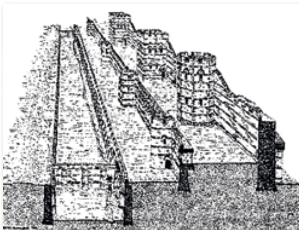
Стіна Феодосія у розрізі. Графічна реконструкція
